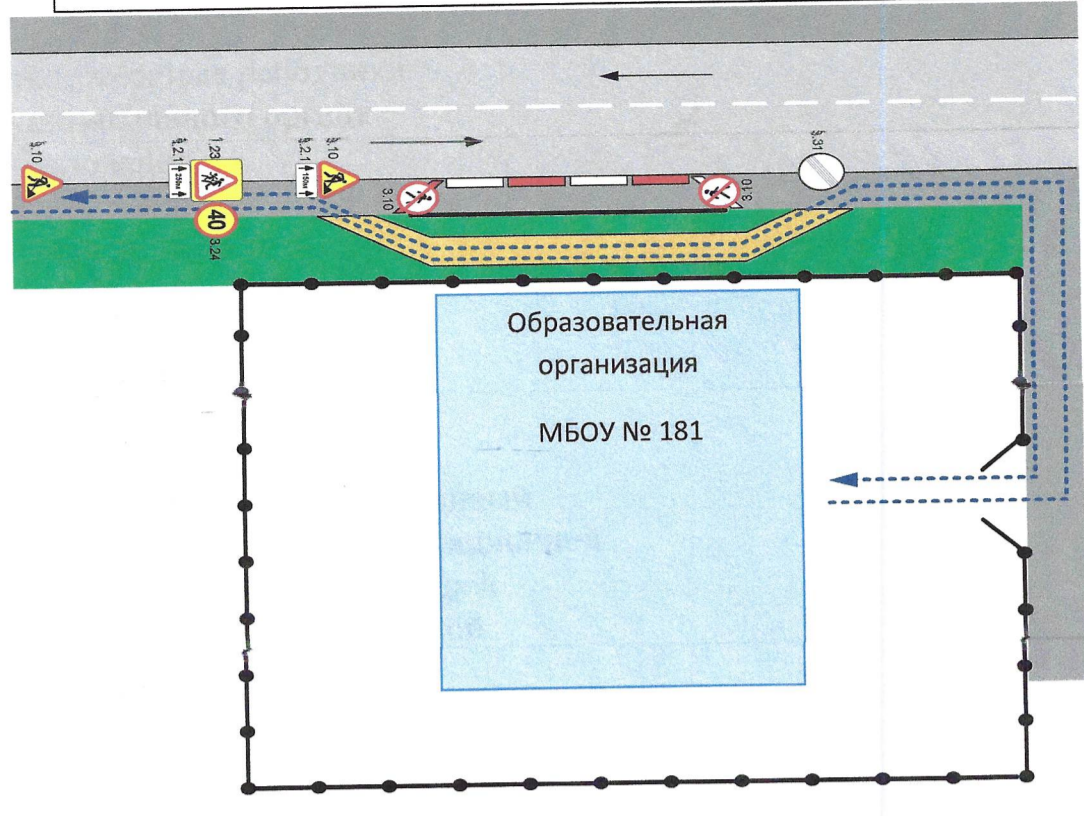
Схема пути движения транспортных средств и детей при проведении дорожных ремонтно-строительных работ вблизи МБОУ № 181.
